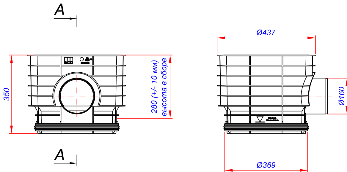
Разрез А-А
